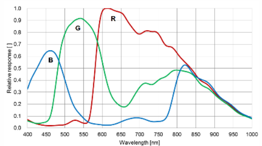
MV-CH089-10UC 量子效率
